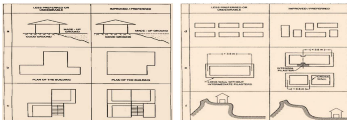
प्लेट 3: सुरक्षित भवनों के योजना और निर्माण के लिए कुछ चित्रण (बीआईएस के एनबीसी से लिया गया)
