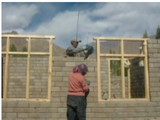
प्लेट 6: ल्हासा में घर: स्थिरीकरण करने वाली सामग्रियों जैसे सीमेंट/चूना का उपयोग करके स्थानीय मिट्टी से निर्मित आवास
